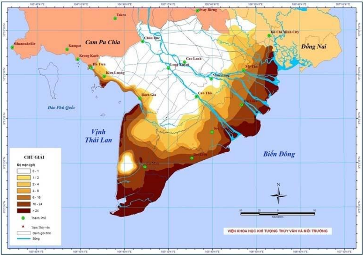
Figure 8 : Gradient de salinité de la nappe phréatique dans le bas delta du Mékong : 0 à 24 g/l (source : Vietnam Times)
