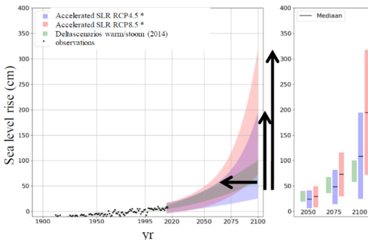
Figure 6 : Hypothèses d'évolution du niveau moyen de la mer (Le Bars et al. , 2017)
