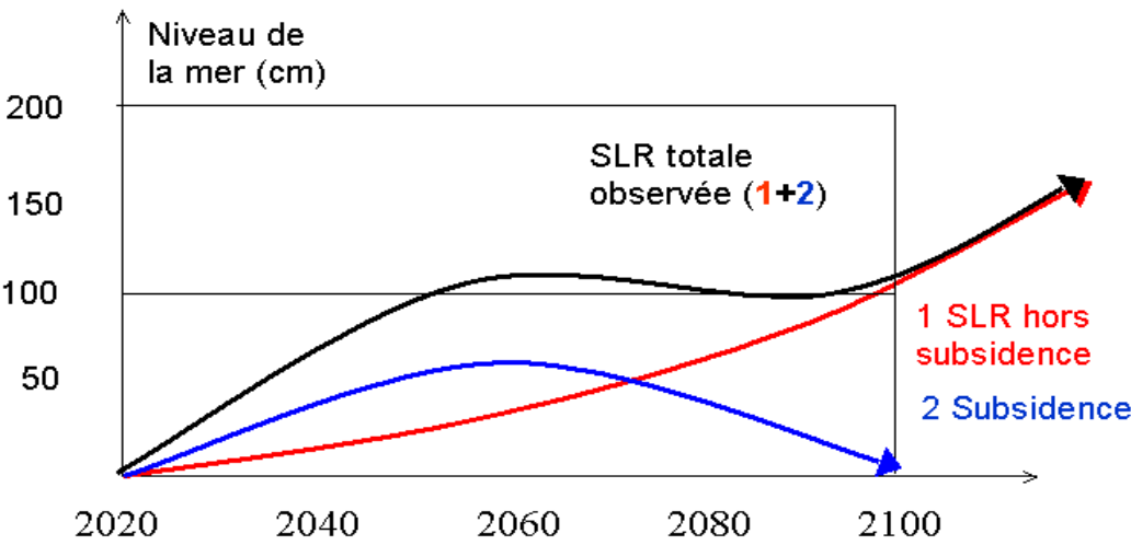
Figure 9 : Schéma d'évolution possible de la hausse du niveau de la mer (Sea level rise, SLR) observée dans les deltas vietnamiens sous les deux hypothèses (1) SLR moyen (+100 cm) et (2) subsidence maîtrisée en 2100
