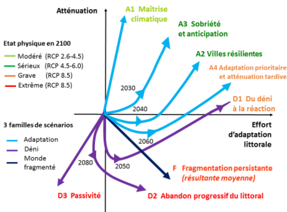
Figure 10 : Schéma de positionnement des huit scénarios selon l'effort d'adaptation littorale et l'atténuation globale
